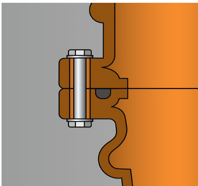
Рисунок: Правильная установка
