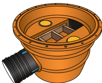
Рисунок: Установка распорок
