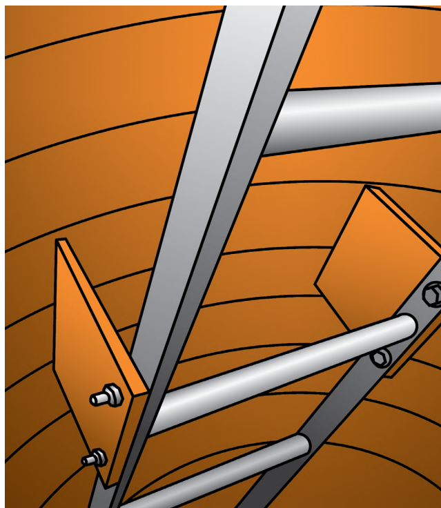
Рисунок: Установка лестницы
