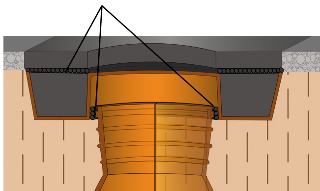
Рисунок: Герметизация каболкой расстояния между ФБ и КП
