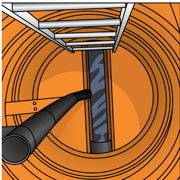
Рисунок: Установка перепадного устройства
