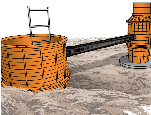
Рисунок: Подключение высотных врезок
