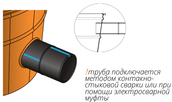
Рисунок: Коннектор РЕ для ПНД и ПВХ труб
