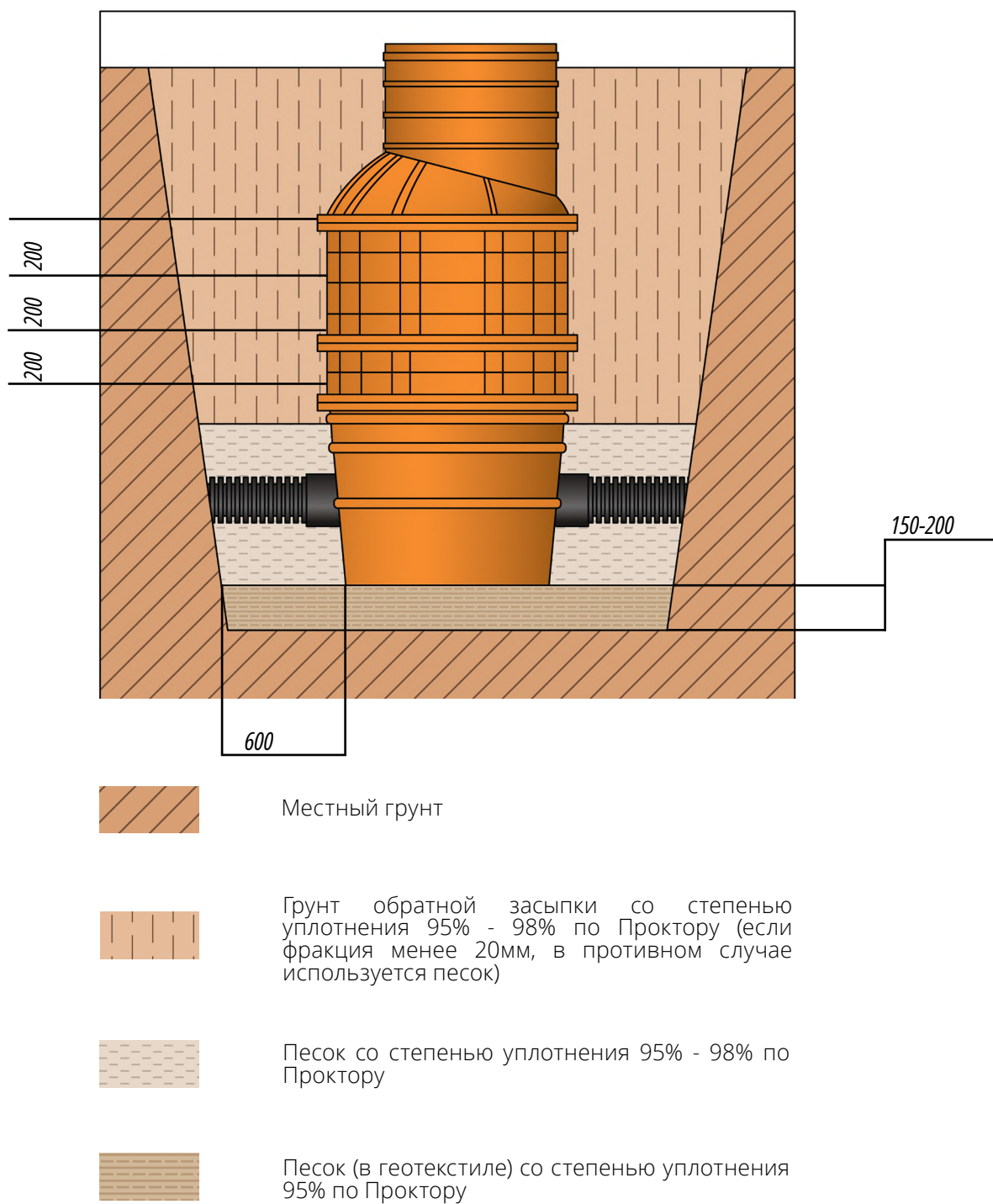
Рисунок: Послойная засыпка и трамбовка
