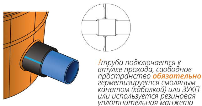
Рисунок: Втулка прохода для ПНД, чугунных труб и др.
