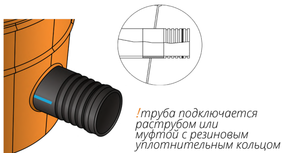
Рисунок: Коннектор IN для гофрированных труб
